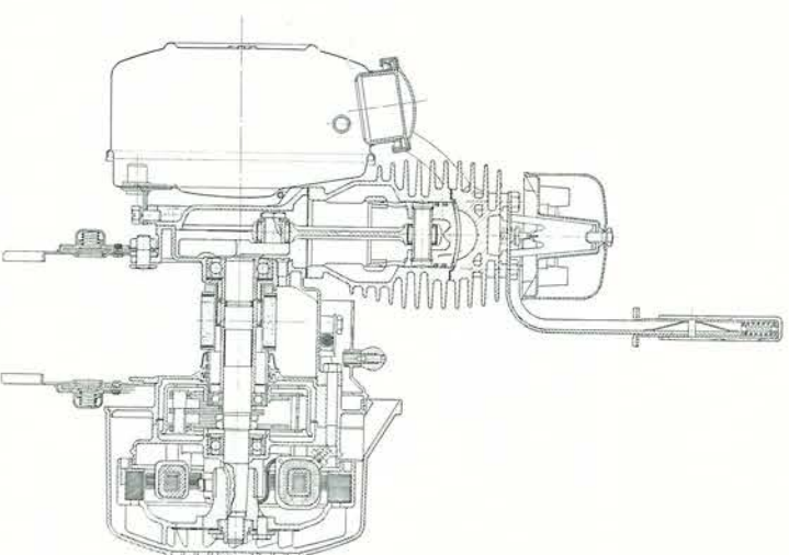
DOORSNEDE SOLEX-MOTOR
