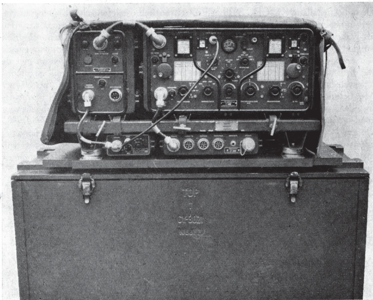
Fig. 1 Radio-installatie KL/GRC-3030, hoofdonderdelen
