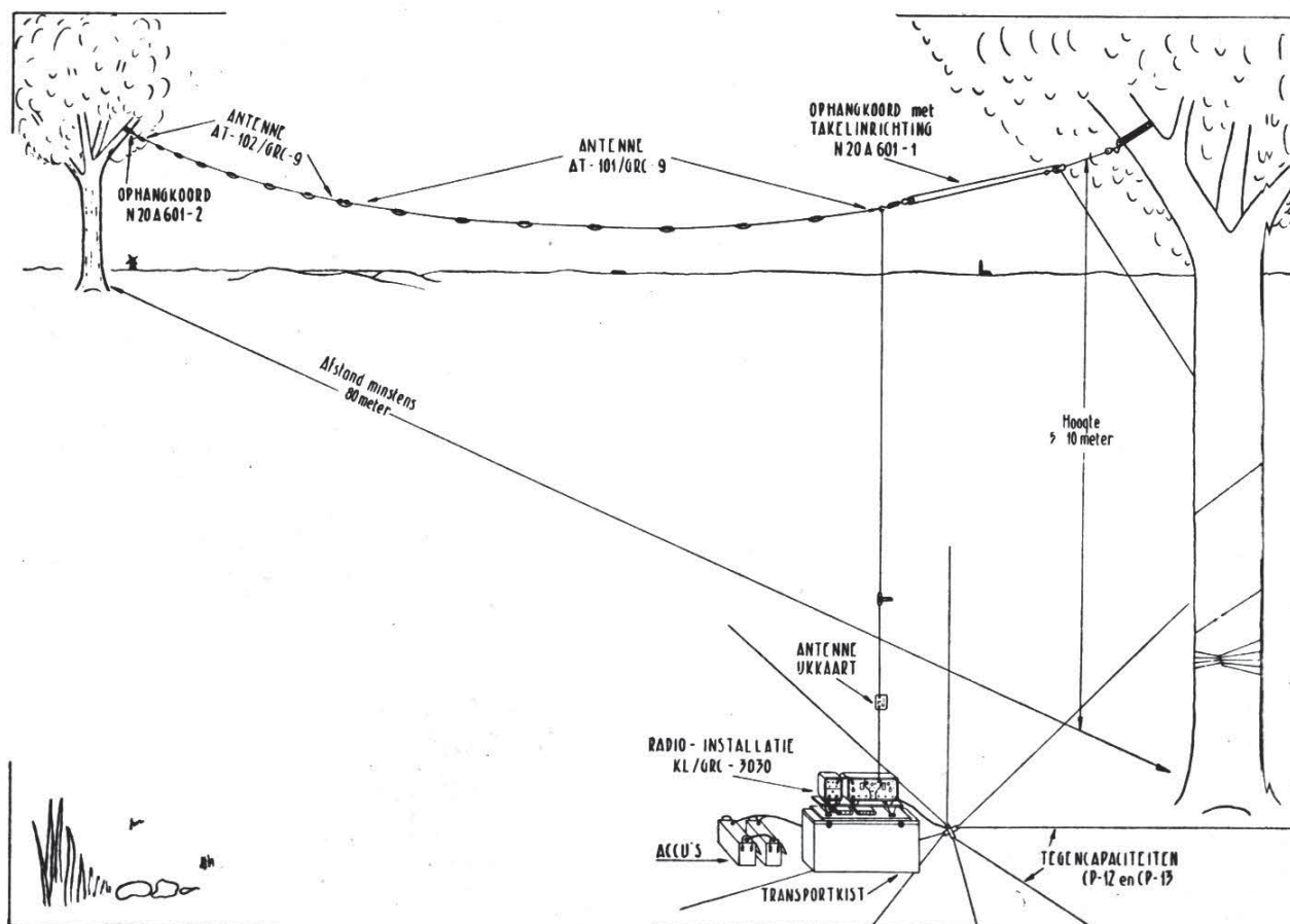
Fig. 8 Het spannen van de draadantenne
