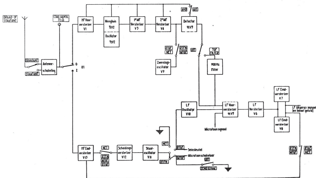
Fig. 9 Zend-ontvanger RT-3030/GRC-3030, blokschema
