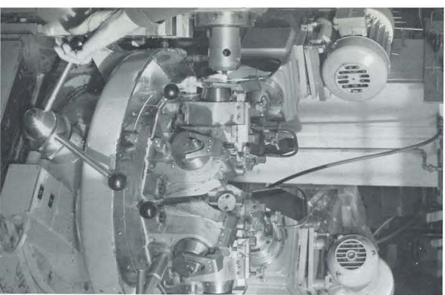
Meerzijdige, automatische kottermachine met draaitafel voor het bewerken van Solex-motoronderdelen.
