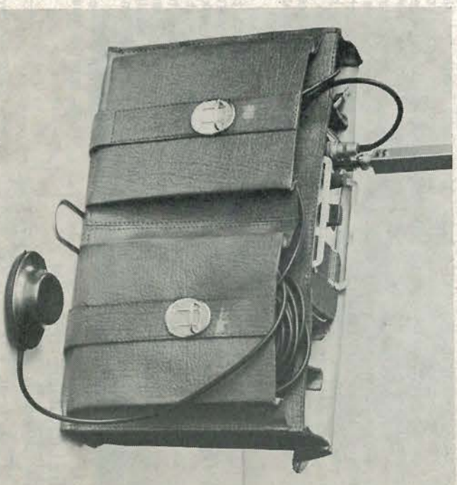
De marifoon in tas, zoals de loods hem meeneemt. Door de uitkapbare voetbeugel kan het geheel rechtop staan.
