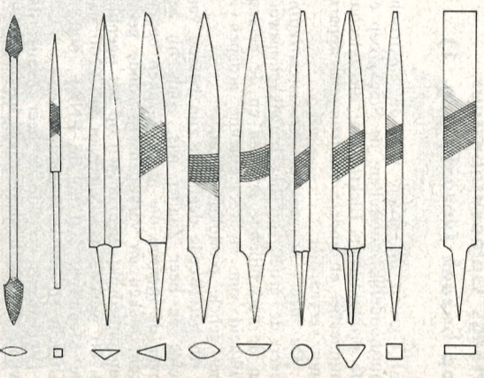
7. Viltvormen en benamingen; van boven naar beneden blokvijl, vierkante vijl, driekante vijl, ronde vijl of rattestaart, halfronde vijl, tongvijl, mesvijl, baretvijl, steelvijl en vormvijl.
