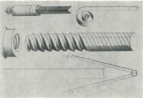
5. Verspanning van schroefdraad met de driekante vijl (1565).
