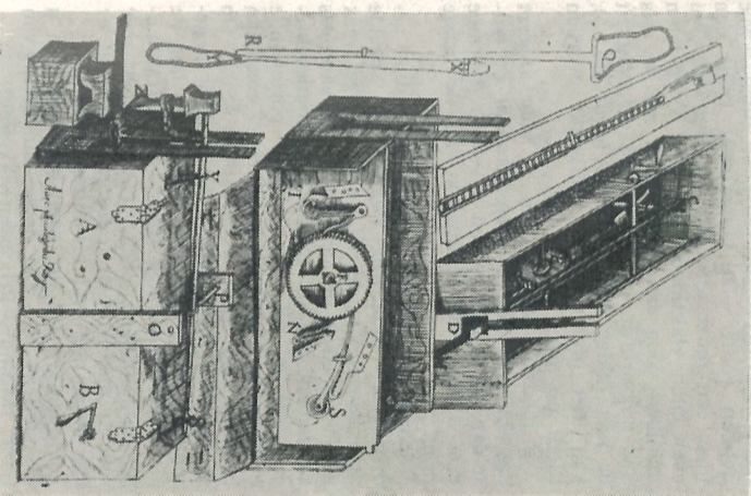
12. Kapwerkting van Jousse.
