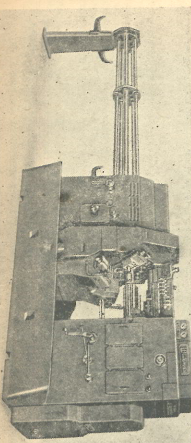
Wickman 5-splijtige automaat
