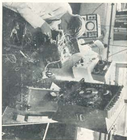
Transistor-meetapparatuur
