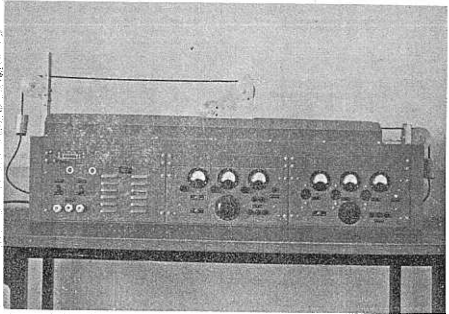
SNOERENFIETS een doeltreffend meetapparaat
