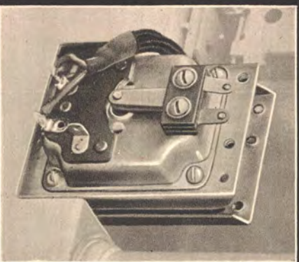
Motor KY 178-179: Deze kleine elektrische motor stelt voor U af
