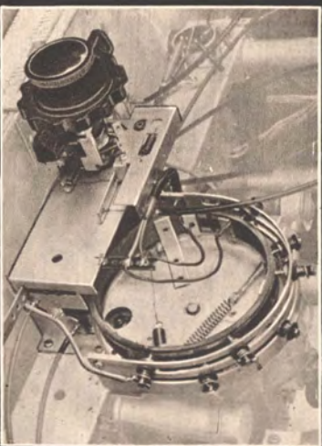
Afstemknop en trommel KY 178-179: De hersenen, die de automatische afstemming commanderen
