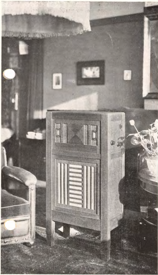
ERRES K.Y. 112, EEN VIER-LAMPSWISSEL- STROOM TOESTEL MET INGEBOUWDE ELECTRO-DYNAMISCHEN LUIDSPREKER f 325.--.
