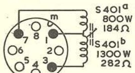
Horizontale blokkerings trafo GK 564 97
