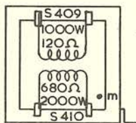
Vert. blokkeringstrafa GK 512 95
