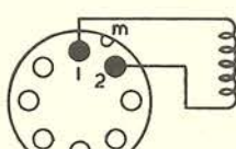
HF Smoorspoel (geluid) GK 564 94
