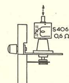
Horizontale breedteregelaar GK 565 21
