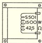
Smoorspoel GK 550 50
