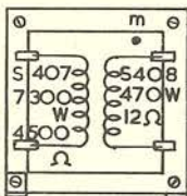
Vert. uitgangstrafa GK 512 93
