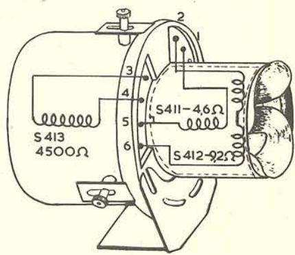
Deflectie-juk GK 565 22
