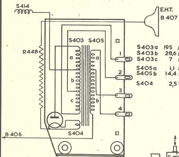
Horizontale uitgangstrafa GK 512 98
