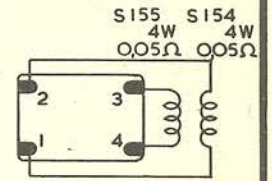
Antennespoel GK 565 24
