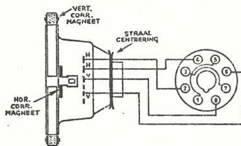
DEFLECTIE JUK DEFLECTION YOKE ABLENKEINHEIT AT 1009/02
