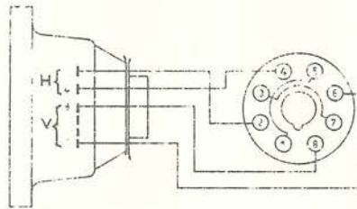
DEFLECTIE JOEK DEFLECTION YOKE ABLENKEINHEIT AT 1009/02
