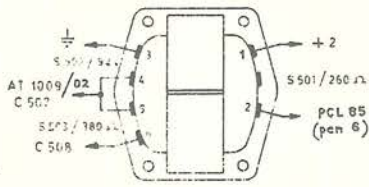
RADIOUITGANGS TRAFU FRAME OUTPUT TRANSF. BILDAUSG. ÜBERTRAGER AT 1009/02
