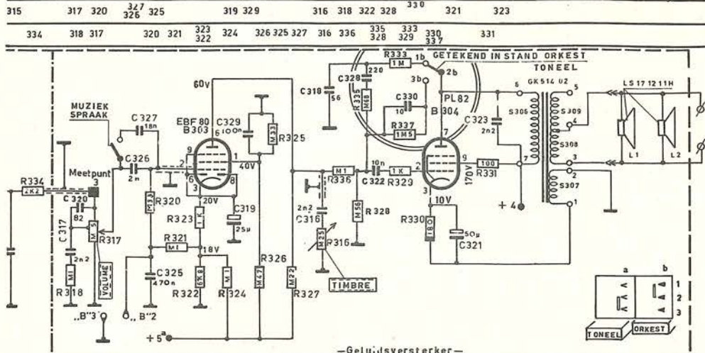
-Geluidsversterker-
