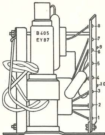
Lijn Uitgangstransformator BT 541
