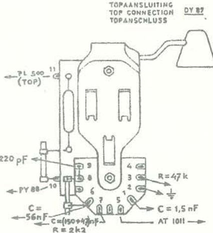
LIJNUITGANGS TRAFU LINE OUTPUT TRANSF. ZEILENAUSG. ÜBERTRAGER AT 2023 50 051 709
