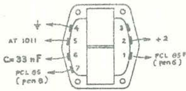
RASTERUITGANGS TRAFU FRAME OUTPUT TRANSF. BILDAUSG. ÜBERTRAGER AT 1011 50 051 708
