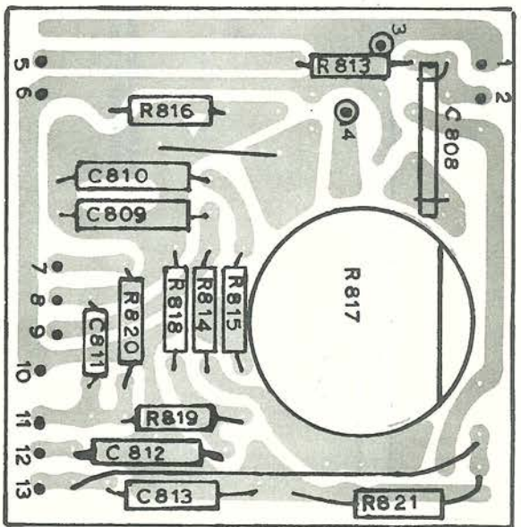
POTENTIOMETERPLAAT PLAQUE DE POTENTIOMÈTRE
