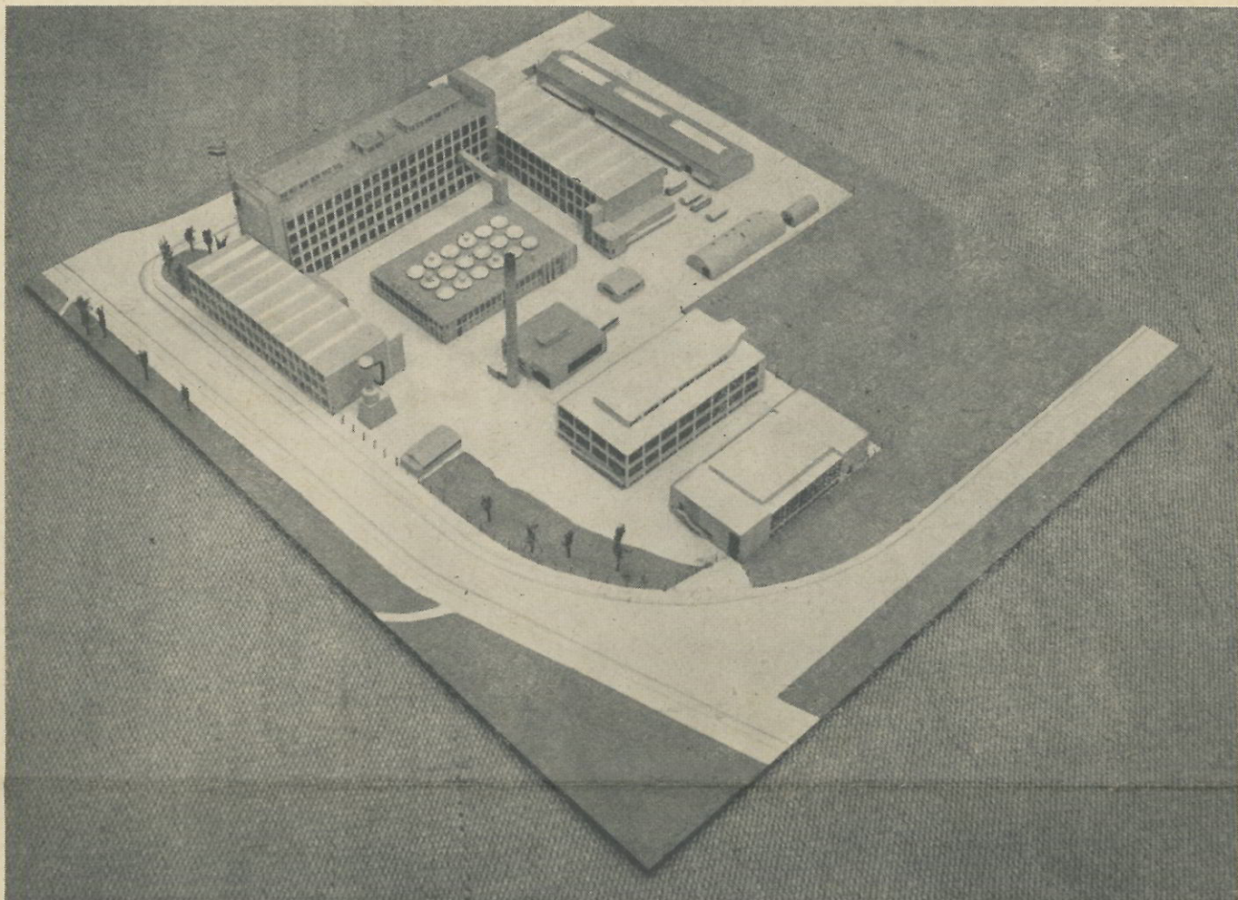
Luchtfoto van de maquette van het fabriekskomplex den Haag, zoals dat zal zijn na gereedkoming van het nieuwe fabrieksgebouw en het personeelsgebouw. De foto is genomen van uit het gezichtspunt: bocht Regulusweg. Alle maten zijn op schaal.
