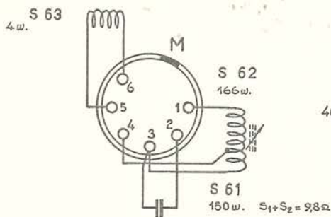
MF.SPOEL III GK 563 76
