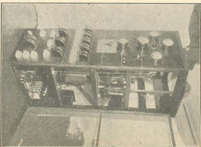
Het hoofdpaneel van den amateurzender op den Radio-Salon.
